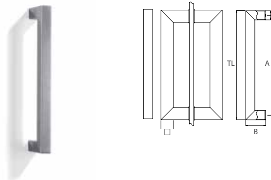
Bohrlochachse A
