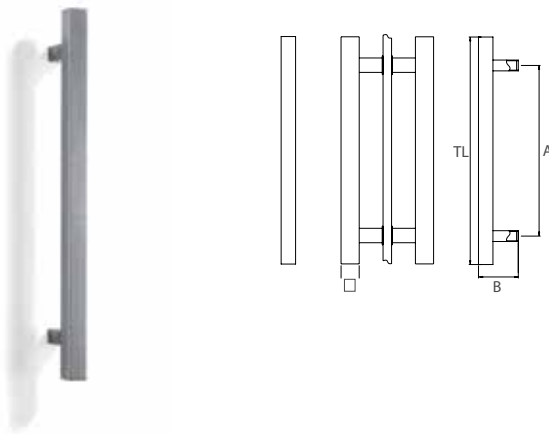
Bohrlochachse A
